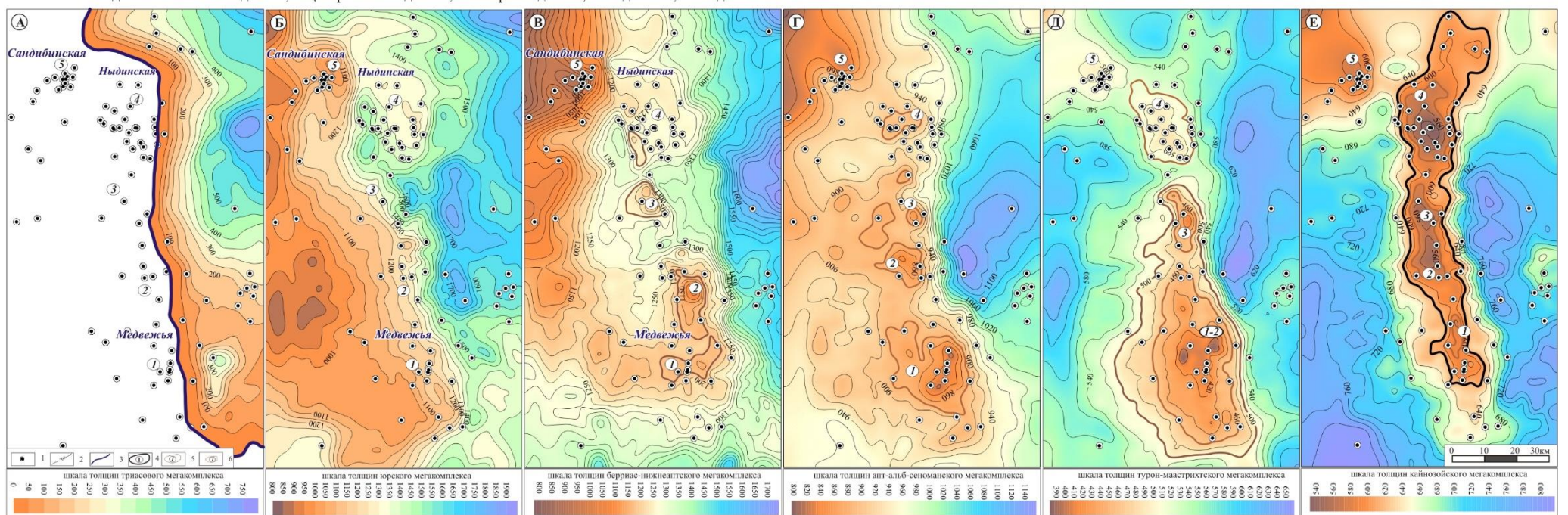
Рисунок 8 - Карты изопакит триасового (А), юрского (Б), берриас-нижнеаптского/ неокомского (В), апт-альб-сенонанского (Г), турон-маастрихтского (Д) и кайнозойского (Е) сейсмогеологических мегакомплексов Условные обозначения: 1-скважины, 2-изопакиты комплексов, 3-зона распространения тампейской серии триаса, 4- контур Медвежьего мезовала, 5-контур Медвежьего вала, 6-локальные поднятия: 1-Южно-Медвежье, 2-Центрально-Медвежье, 3-Северо-Медвежье, 4-Ныдинское, 5-Сандыбинское
