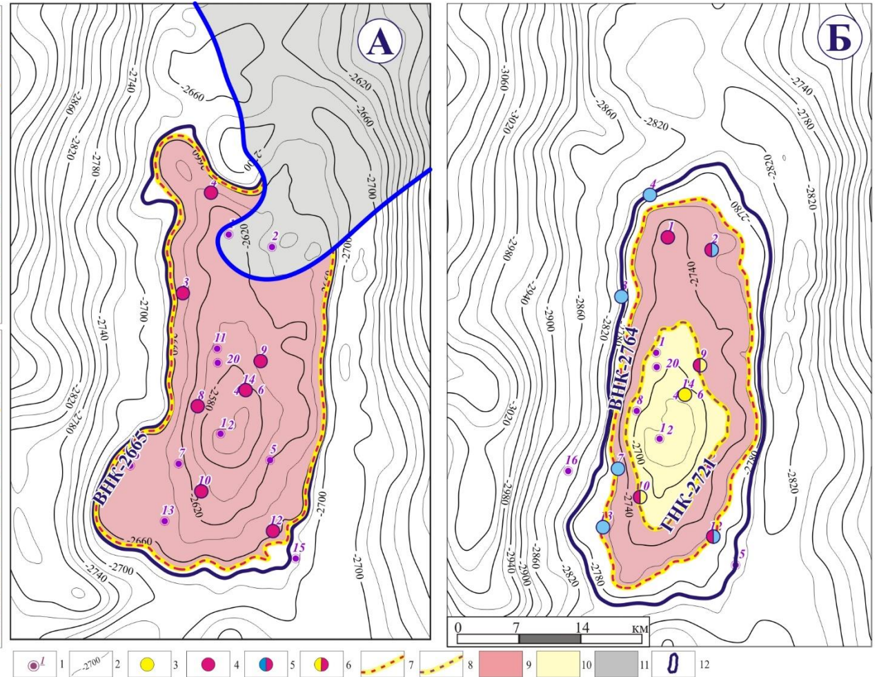
Рисунок 16 - Модель нефтяной залежи пласта Нх-I (А) и газонефтяной залежи пластов Нх-III-IV (Б) Ванкорского месторождения Условные обозначения: 1-скважины, 2-изогипсы; скважины с притоками: 3-газа, 4-нефти, 5-нефти и воды, 6-нефти и газа; 7-водонефтяной контакт, 8-газонефтяной контакт, 9-нефтяная залежь, 10-газовая залежь, 11- зона отсутствия коллектора, 12-контур Ванкорского поднятия
