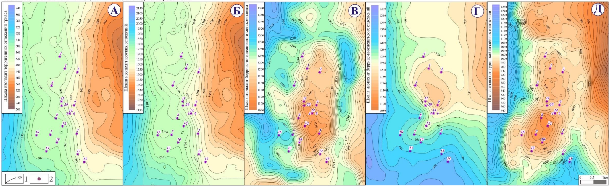
Рисунок 6 - Карты изопакит триасовых (А), юрских (Б), берриас-нижнеаптских /неокомских/ (В), апт-альб-сенонанских (Г) и турон-кайнозойских (Д) отложений (Ванкорское месторождение) Условные обозначения: 1-изопакиты комплексов, 2-скважины
